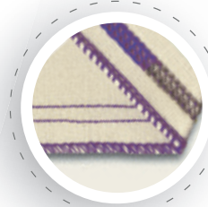
6-Faden Ziernaht 16 mm Rollnaht kombiniert mit Covernaht
